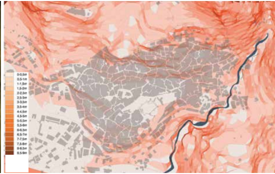
Plànol pluviomètric
