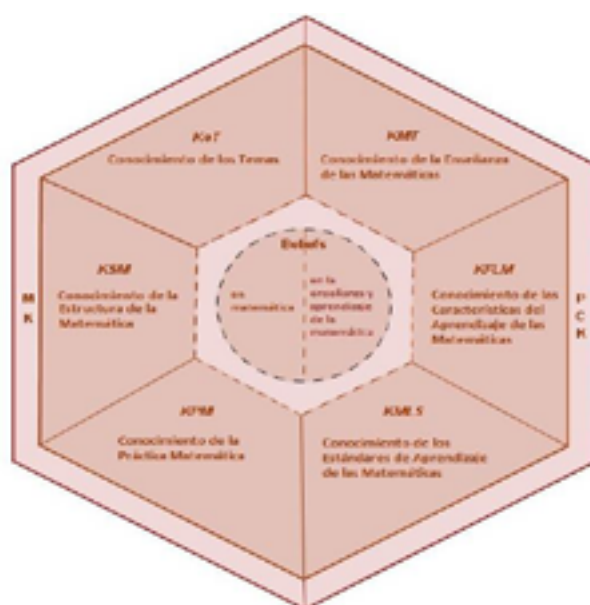
FIGURA 1 MODELO MTSK
